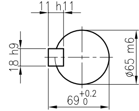
OUTPUT SHAFT (18x11x113)
